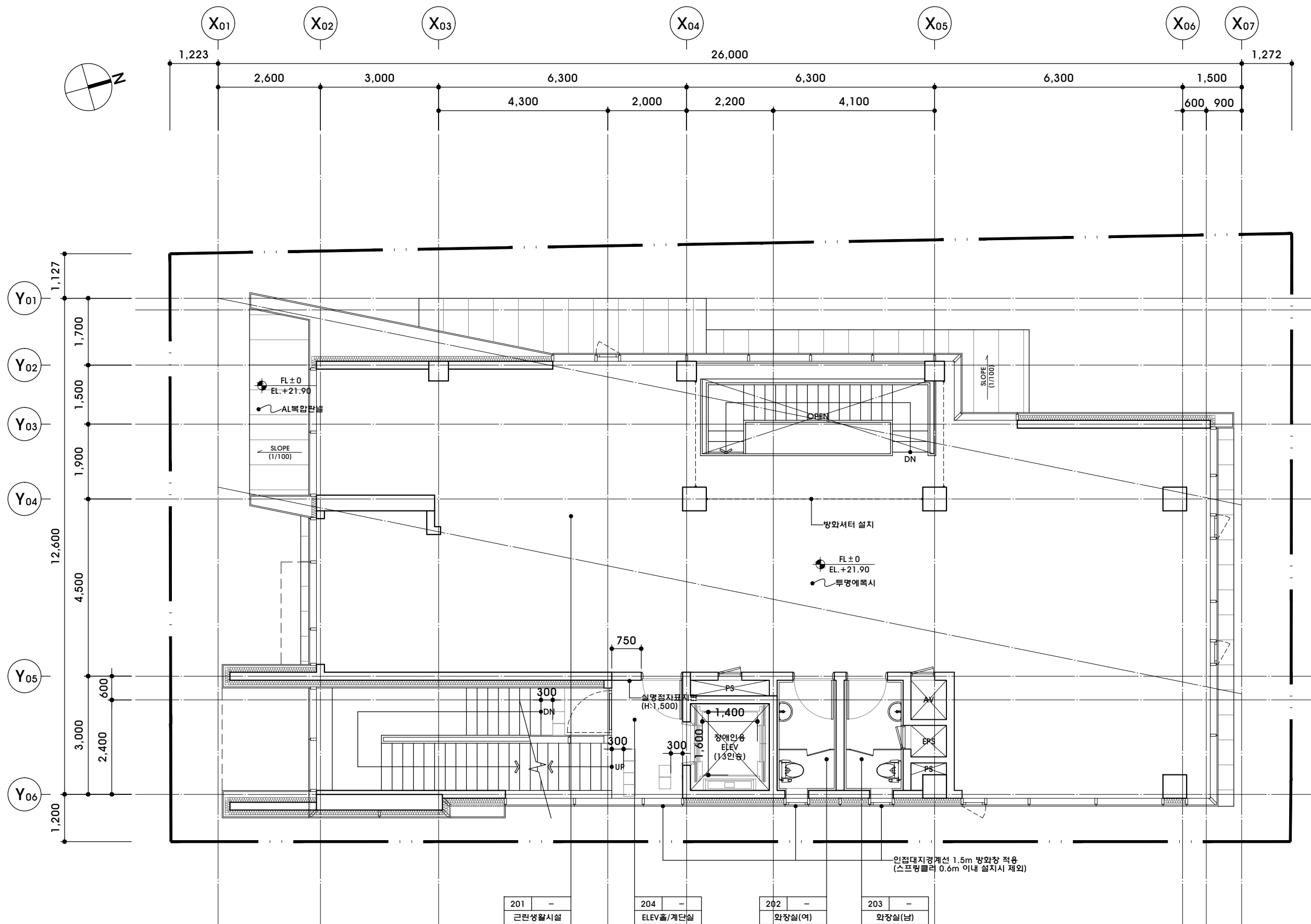
1 A-305 지상2층 평면도 축척 : 1/100
