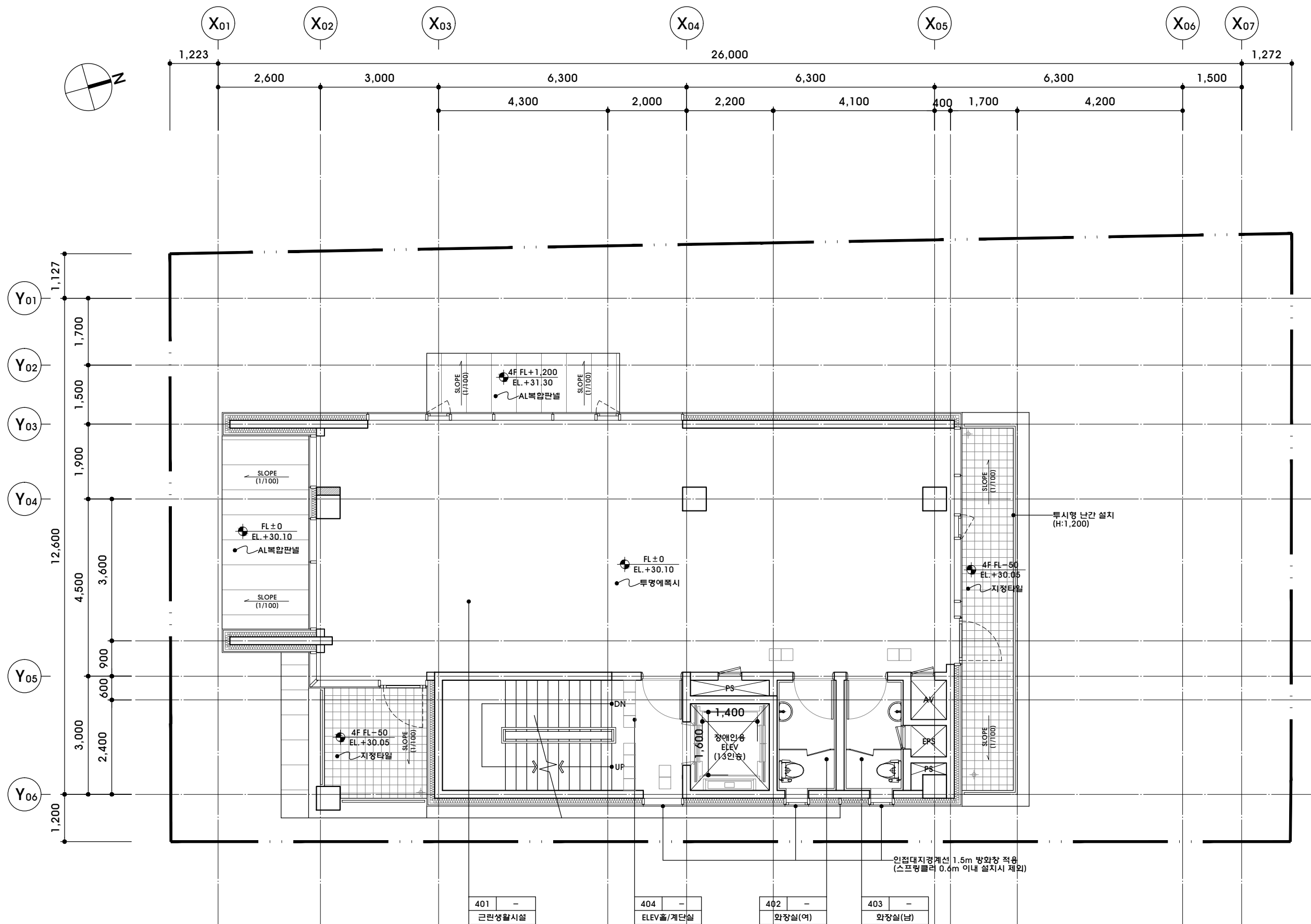
1 A-307 지상4층 평면도 축척 : 1/100
