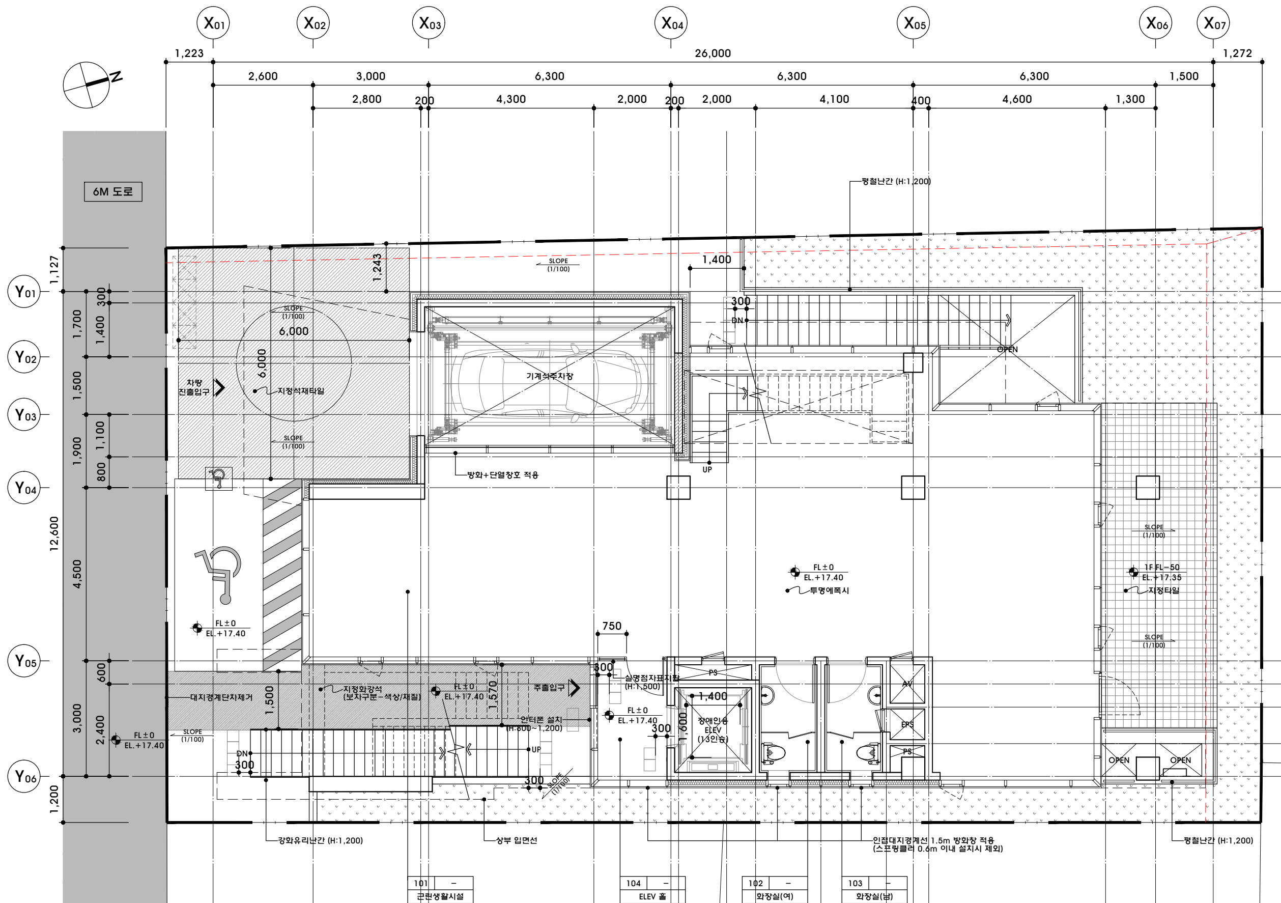
1 A-304 지상1층 평면도 축척 : 1/100
