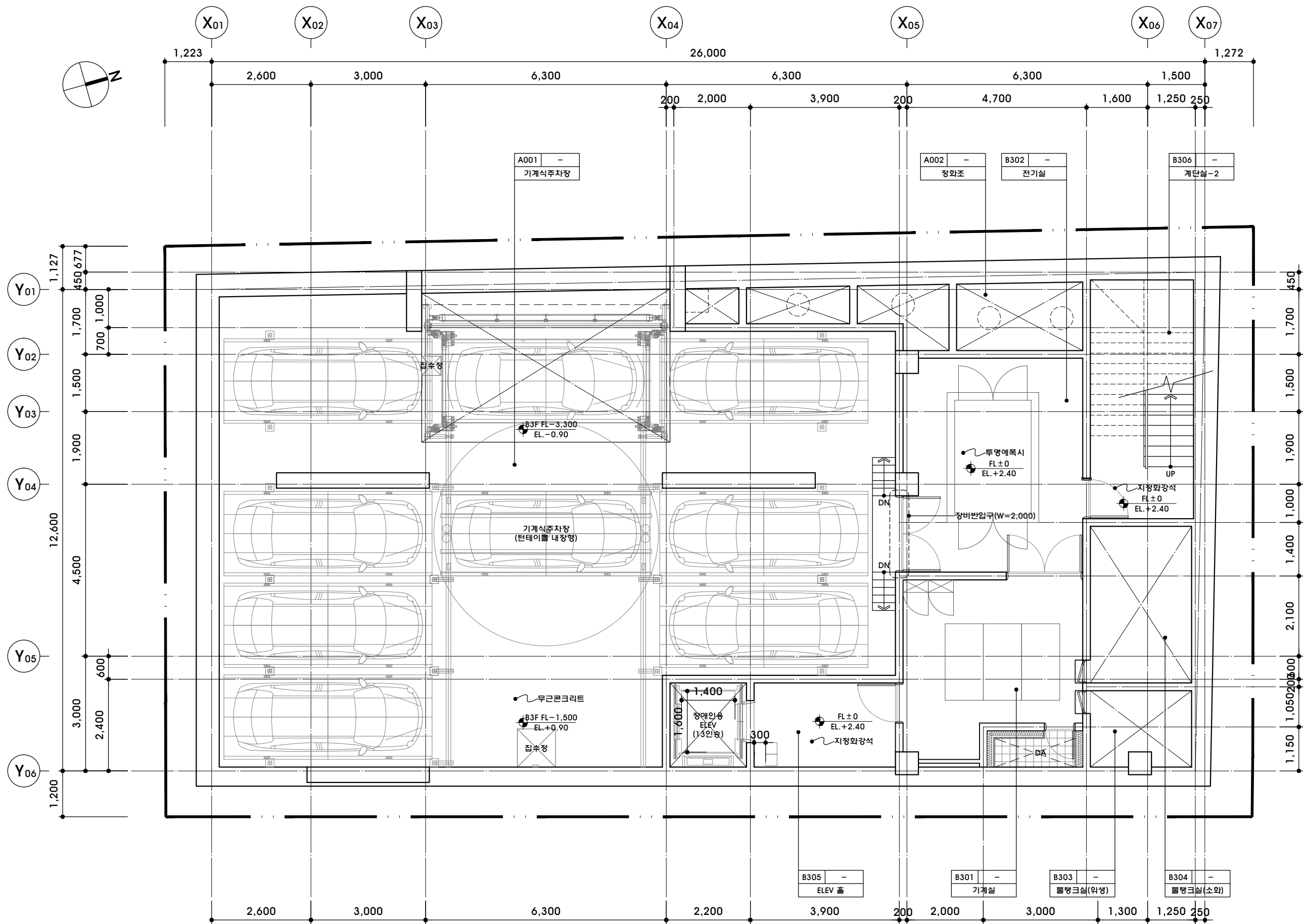
1 지하3층 평면도 축척 : 1/100 A-301
