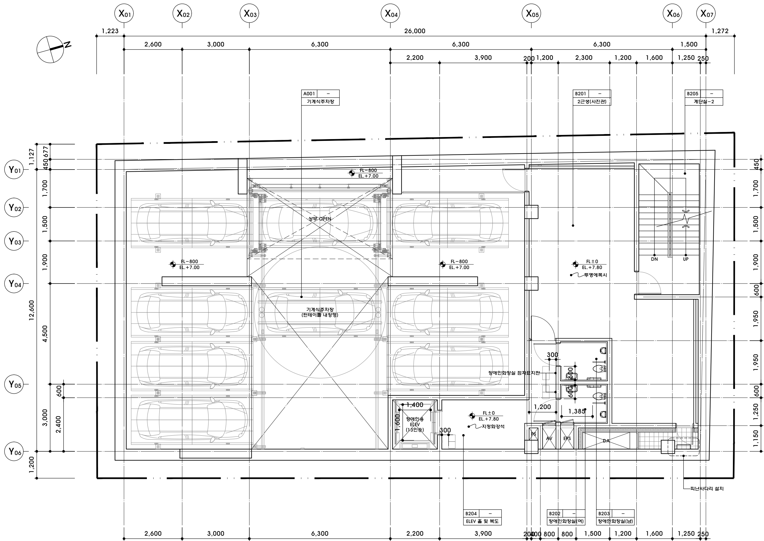
1 지하2층 평면도 축척 : 1/100
